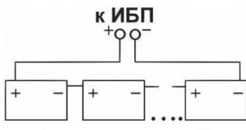
Рисунок 3.5. Подключение внешних батарей к ИБП версии Н
